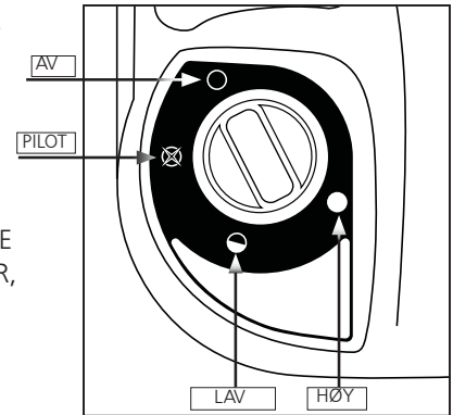
Figur 1: Kontrollknapp
