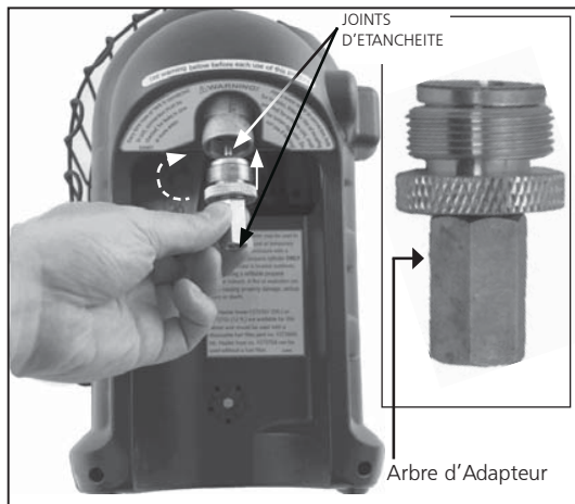
Figure 4 : "Adaptateur de Butane"
