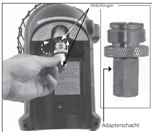
Afbeelding 4: "Butaanadapter"
