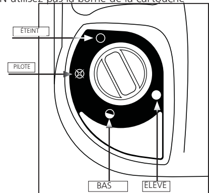
Figure 1 : Bouton de commande
