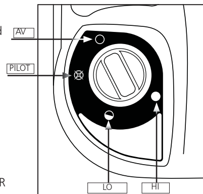
Figur 1: Reglagevredet
