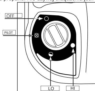
Rysunek 1: Pokrętło
