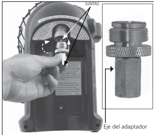
Figura 4: "Adaptador de butano"
