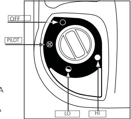
Kuva 1: Säätönappi
