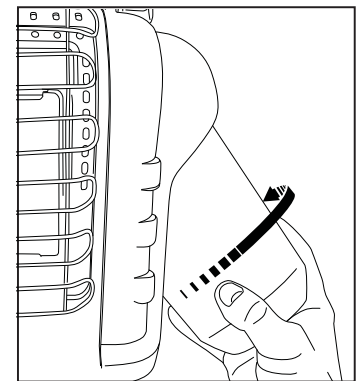
Afbeelding 2: Gastank aansluiten
