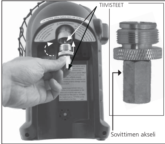
Kuva 4: "Butaanisovitintä"
