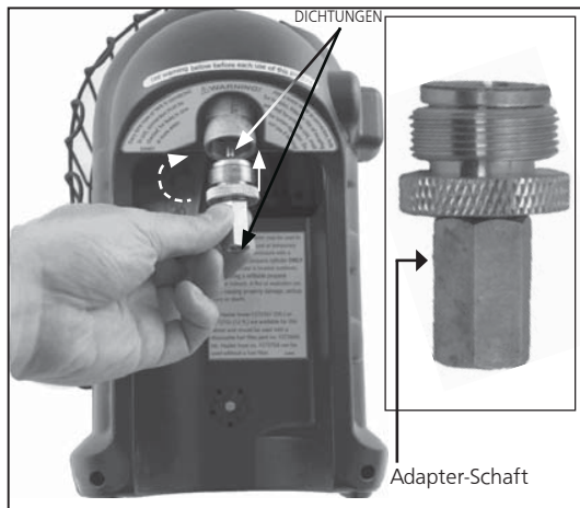
Abbildung 4: „Butan Adapter“
