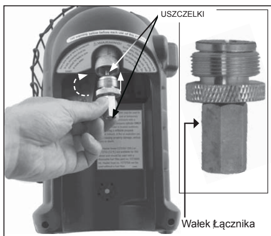
Rysunek 4: "Łącznik Butanu".
